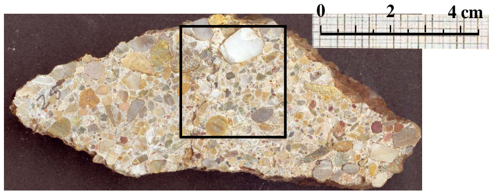
09_1 : Micro conglomérat polygénique à éléments carbonatés (x 1)
